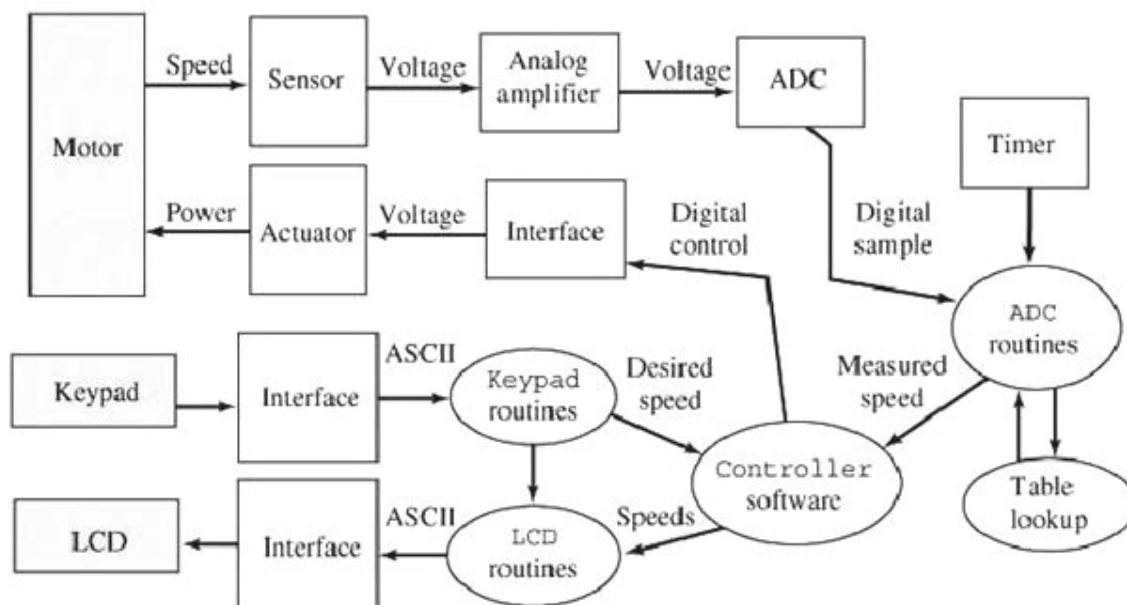
Hình 2.2 Sơ đồ tổng quát của một hệ thống điều khiển động cơ
