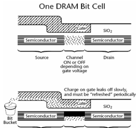
Cấu trúc một phân tử nhớ DRAM
