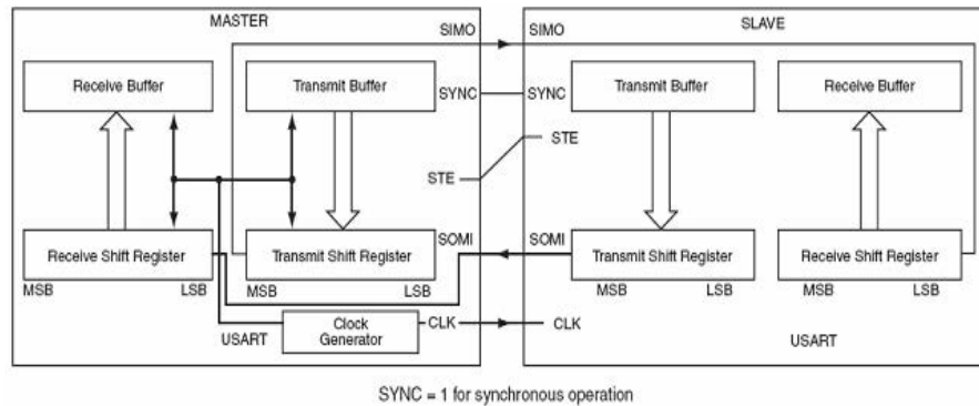
Mode hoạt động truyền thông đồng bộ
