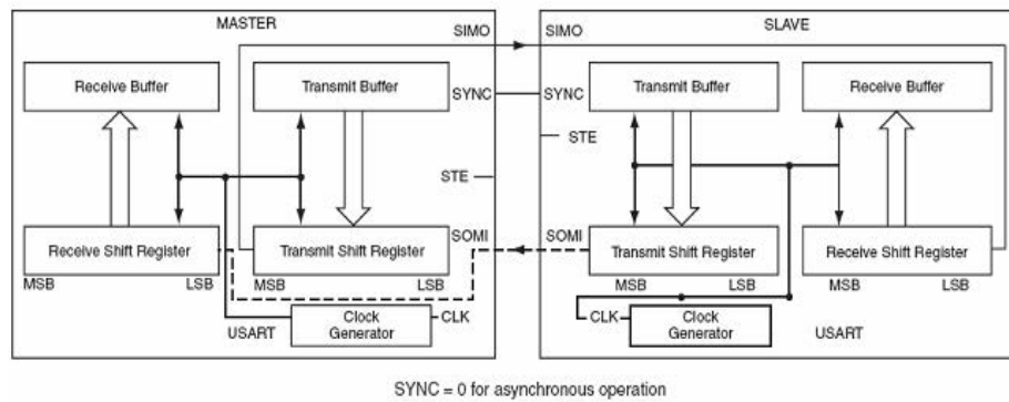
Mode hoạt động truyền thông dị bộ
