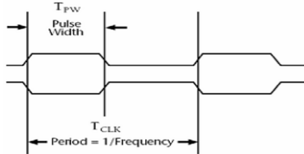
Độ rộng và tần số xung nhịp chuẩn
