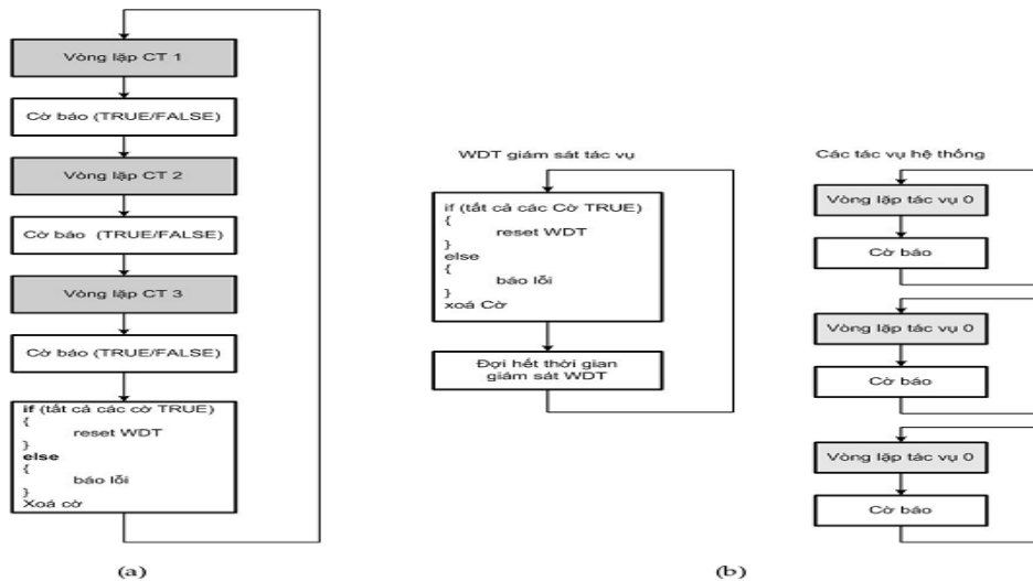
Nguyên lý hoạt động của bộ định thời
