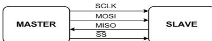
Kết nối nguyên lý truyền thông SPI giữa một Master và Slave
