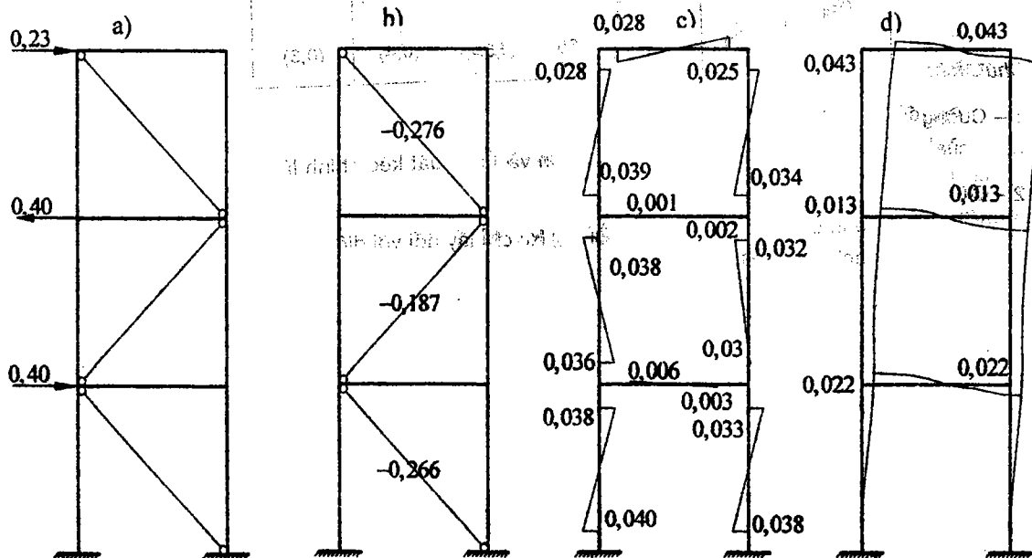
Hình 7.8. Tính toán dạng dao động thứ ba của khung a) Sơ đồ tĩnh; b) Lực dọc trong dải khối xây chèn tương đương, T; c) Mômen trong khung, Tm; d) Chuyển vị ngang, mm.
