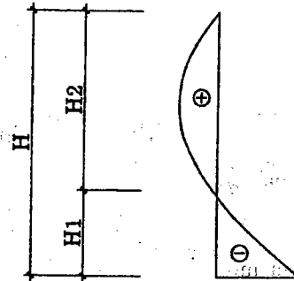
Hình 4.7. Biểu đồ mômen đổi dấu theo chiều cao của cấu kiện chịu nén
