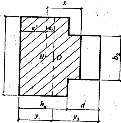
Hình 1. Vùng nén khi độ lệch tâm ở phía cánh
