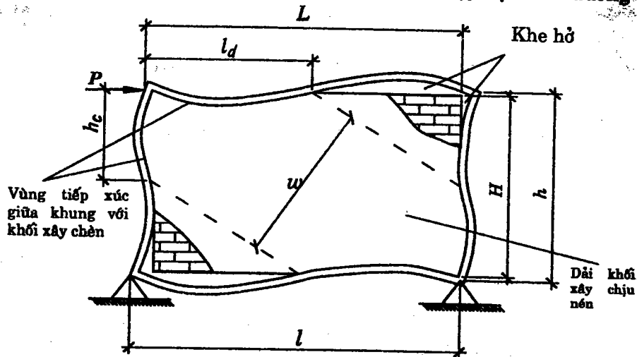
Hình 7.1. Biến dạng của khung BTCT chèn gạch chịu lực ngang
