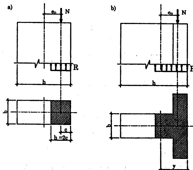
Hình 4.6. Sơ đồ tính toán khối xây chịu nén lệch tâm
