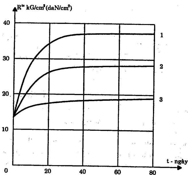
Hình 2.6. Cường độ khối xây theo thời gian 1 - mác vữa 100; 2 - mác vữa 25; 3 - mác vữa 4.
