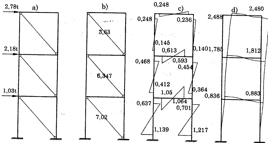
Hình 7.6. Tính toán dạng dao động thứ nhất của khung a) Sơ đồ tính; b) Lực dọc trong dải khối xây chèn tương đương, t; c) Mômen trong khung, tm; d) Chuyển vị ngang, mm.
