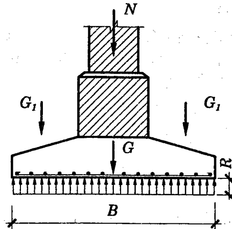
Hình 6.6. Cấu tạo móng mềm
