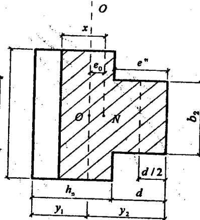
Hình 2. Vùng nén khi độ lệch tâm ở phía sườn
