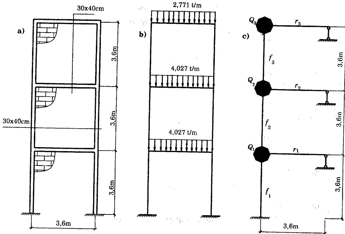
Hình 7.5. Tính khung chèn gạch chịu tải trọng động đất a) Khung với khối xây chèn; b) Tải trọng thẳng đứng; c) Sơ đồ tính
