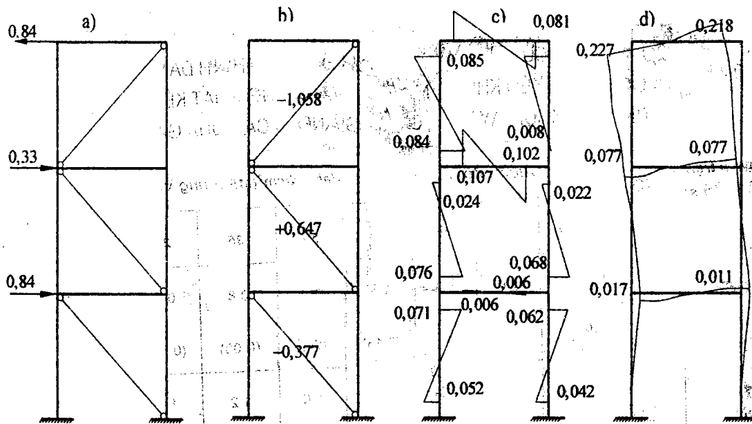
Hình 7.7. Tính toán dạng dao động thứ hai của khung a) Sơ đồ tĩnh; b) Lực dọc trong dải khối xây chèn tương đương, T; c) Mômen trong khung, Tm; d) Chuyển vị ngang, mm.
