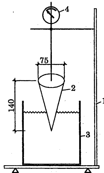
Hình 1.3. Thiết bị đo độ sệt vữa 1- giá đỡ; 2 - quả chùy tiêu chuẩn G=300gam;
