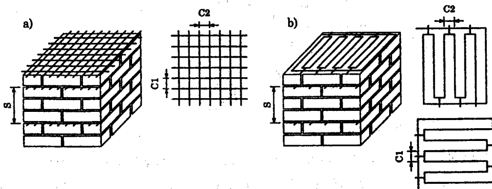
Ảnh 5.1. Gia cường khối xây bằng lưới thép ngang a) Lưới chữ nhật; b) Lưới zíc zắc.
