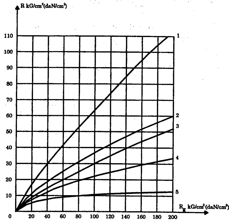
Hình 2.4. Quan hệ giữa cường độ gạch R_g và cường độ khối xây R khi R_g = 25
