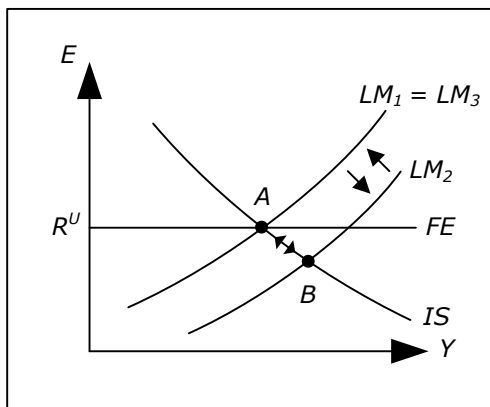
Fig. 16.3: IS-LM-FE.
