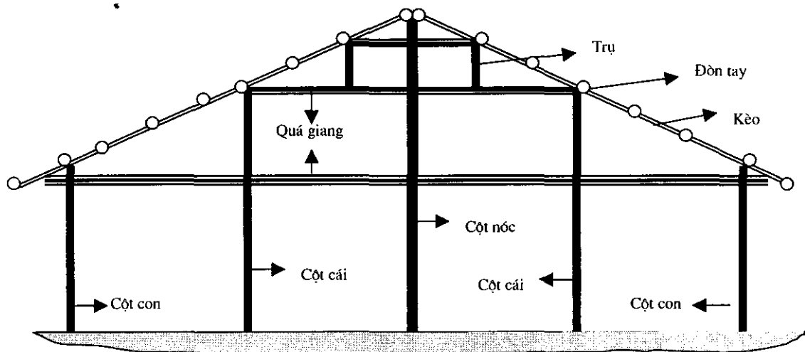
Hình 3: Vì kèo 5 cột
