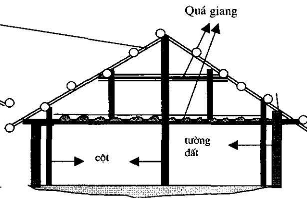
Hình 2: Vì kèo giữa 3 cột (trấn cột cái)
