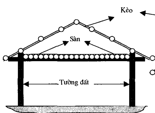
Hình 1: Vì kèo không có cột
