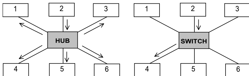
Hình 3.25: Nguyên tắc làm việc của bộ chia và bộ chuyển mạch
