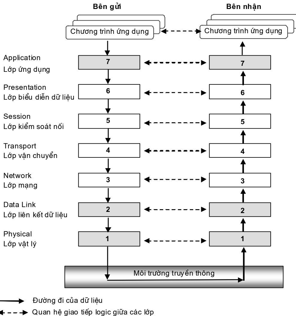
Hình 2.38: Mô hình qui chiếu ISO/OSI
