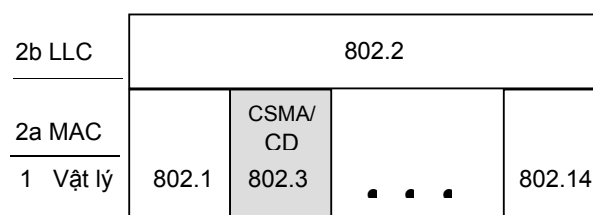
Hình 4.19: Ethernet/IEEE 802.3 trong tập chuẩn IEEE 802
