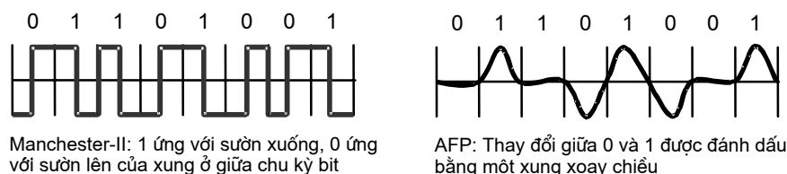
Hình 2.22: Mã hóa bit Manchester-II và AFP
