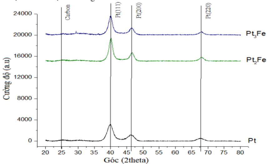
Hình 4. Giản đồ XRD của các mẫu vật liệu nano Pt/C, Pt 2 Fe/C, Pt 3 Fe/C
