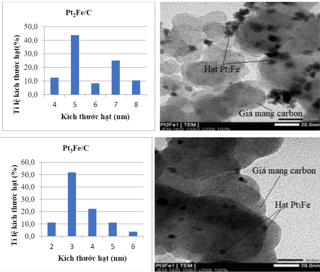
Hình 3. Biểu đồ phân bố kích thước hạt và ảnh TEM của mẫu Pt/VC, Pt 2 Fe/VC, Pt 3 Fe/VC như vậy, từ các mẫu khảo sát đều cho kết quả vật liệu tổng hợp có được kích thước nano từ 2 - 8 nm và sản phẩm tổng hợp vẫn cho thấy có kết tụ đám ở một số vùng đối với mẫu Pt/C, Pt 2 Fe/C, Pt 3 Fe/C. Mẫu Pt 3 Fe/C, Pt/C có kích thước hạt bé hơn mẫu Pt 2 Fe/C như Bảng 1.
