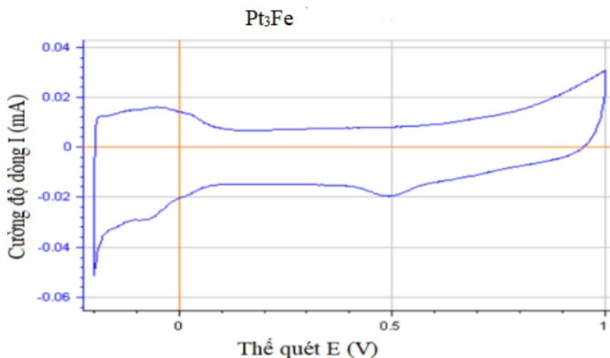
Hình 5. Đường cong CV của các mẫu \text{Pt}_3\text{Fe/C} trong \text{N}_2/0,5\text{ M H}_2\text{SO}_4
